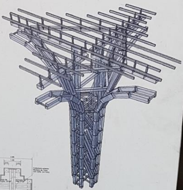
Isometría de estructura de un pilar
