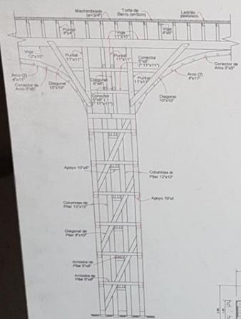
Elevación de un pilar y sistema de techo horizontal sobre él
