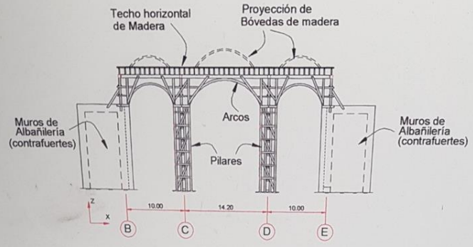
Elevación de los elementos de la estructura
